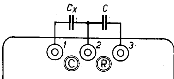
Meten van capaciteiten groter dan 10 \mu\text{F}
