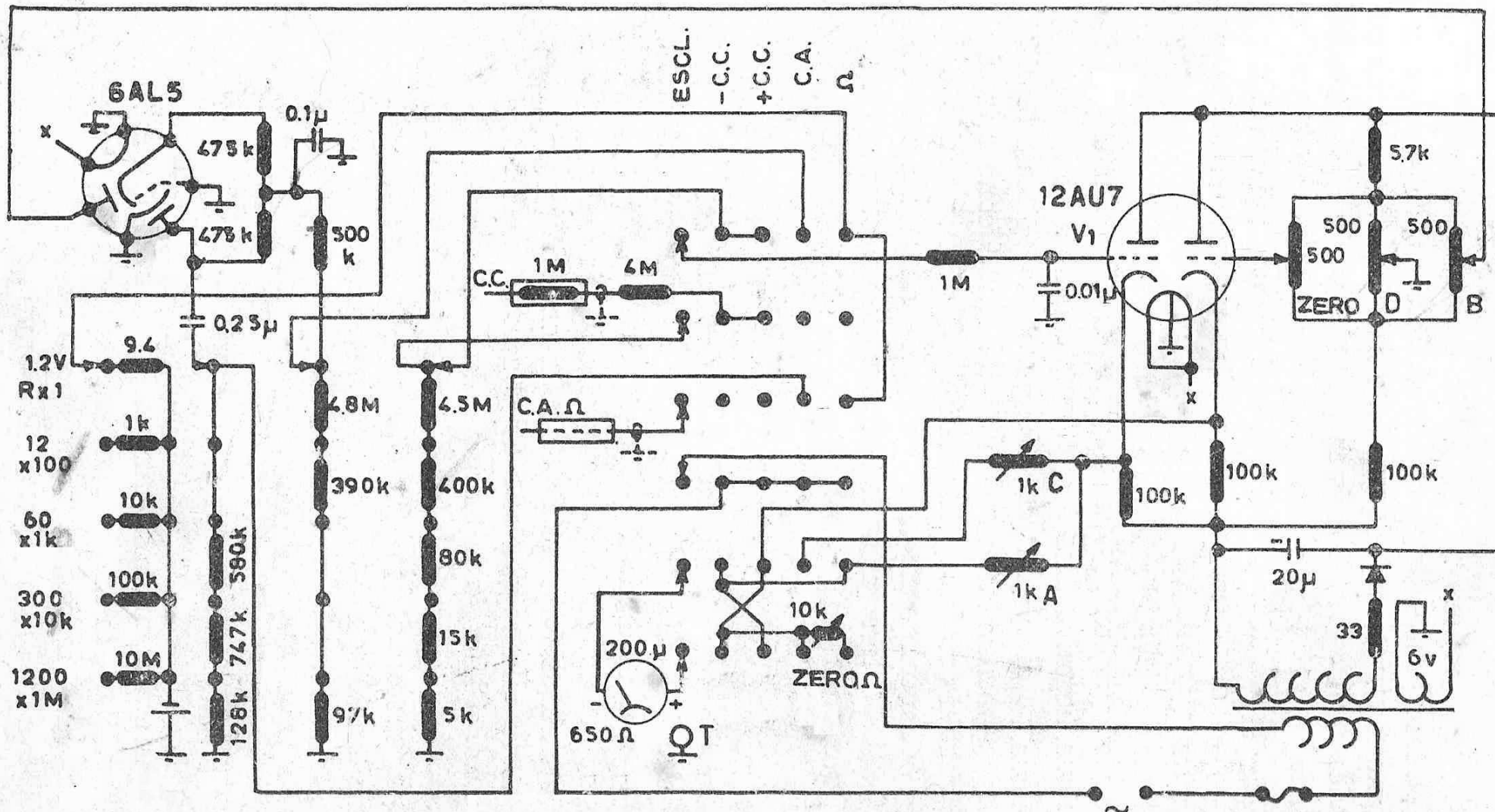
Simpson 303 Voltmeter
