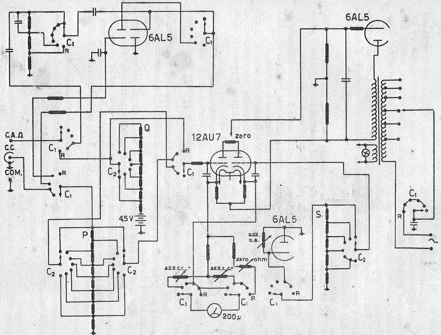
Fig. 72. - Voltmetro elettronico UNA R-122.
