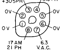
V-6 6V6 GT
