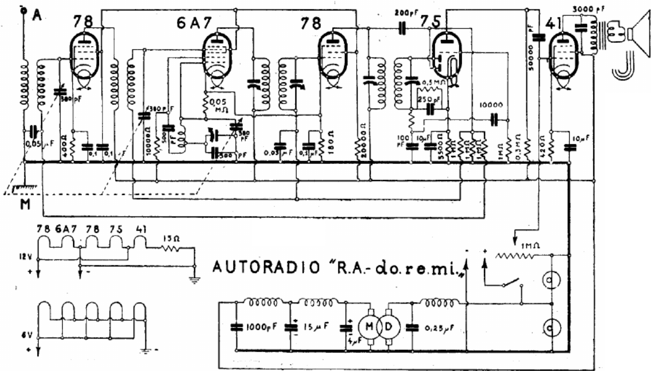
DOLFIN RADIO . MOD. « AUTORADIO DO-RE-MI »
