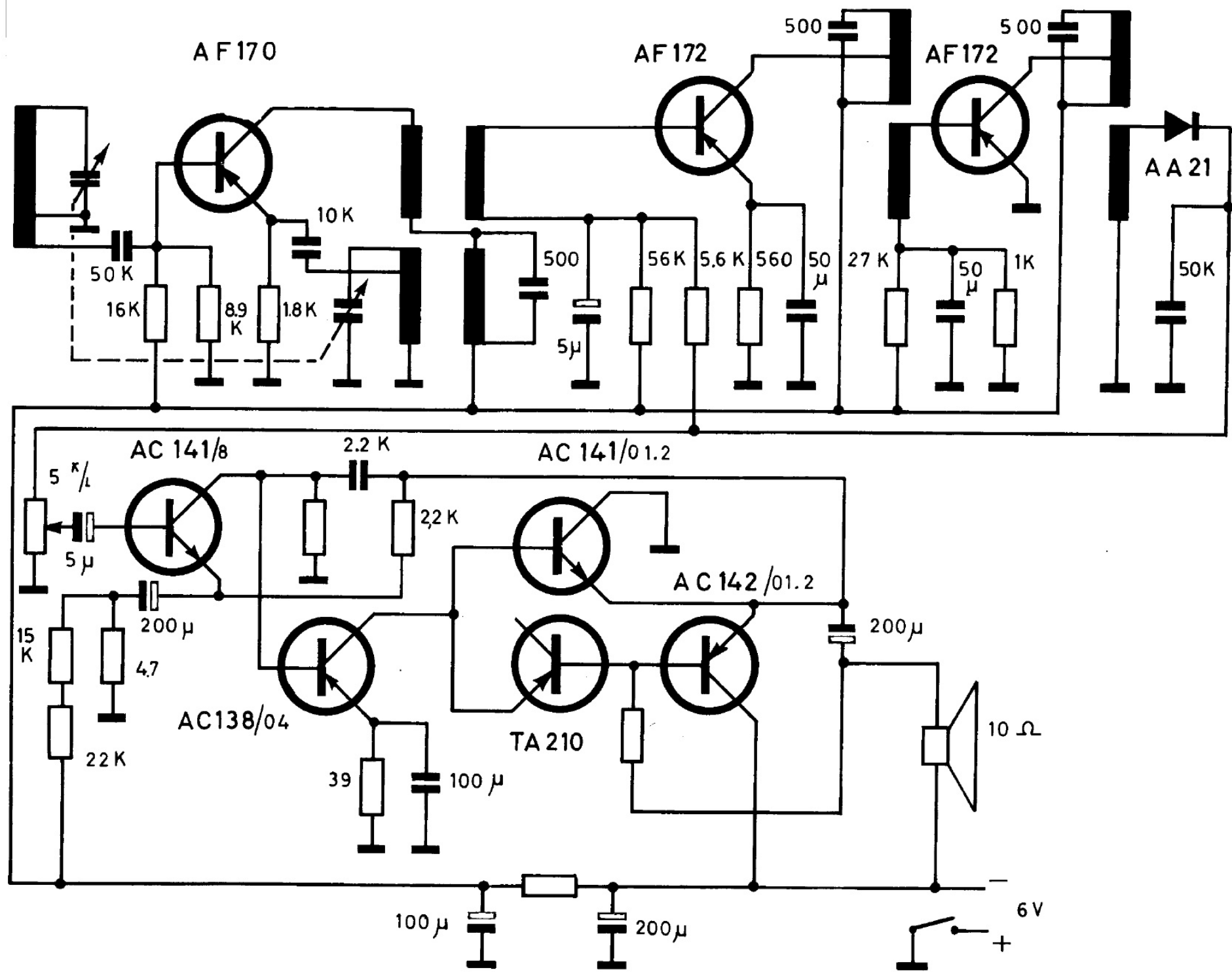
SCHEMA ELETTRICO DEL RARIODICEVITORE G.B.C. AR/28A TERRY BOY
