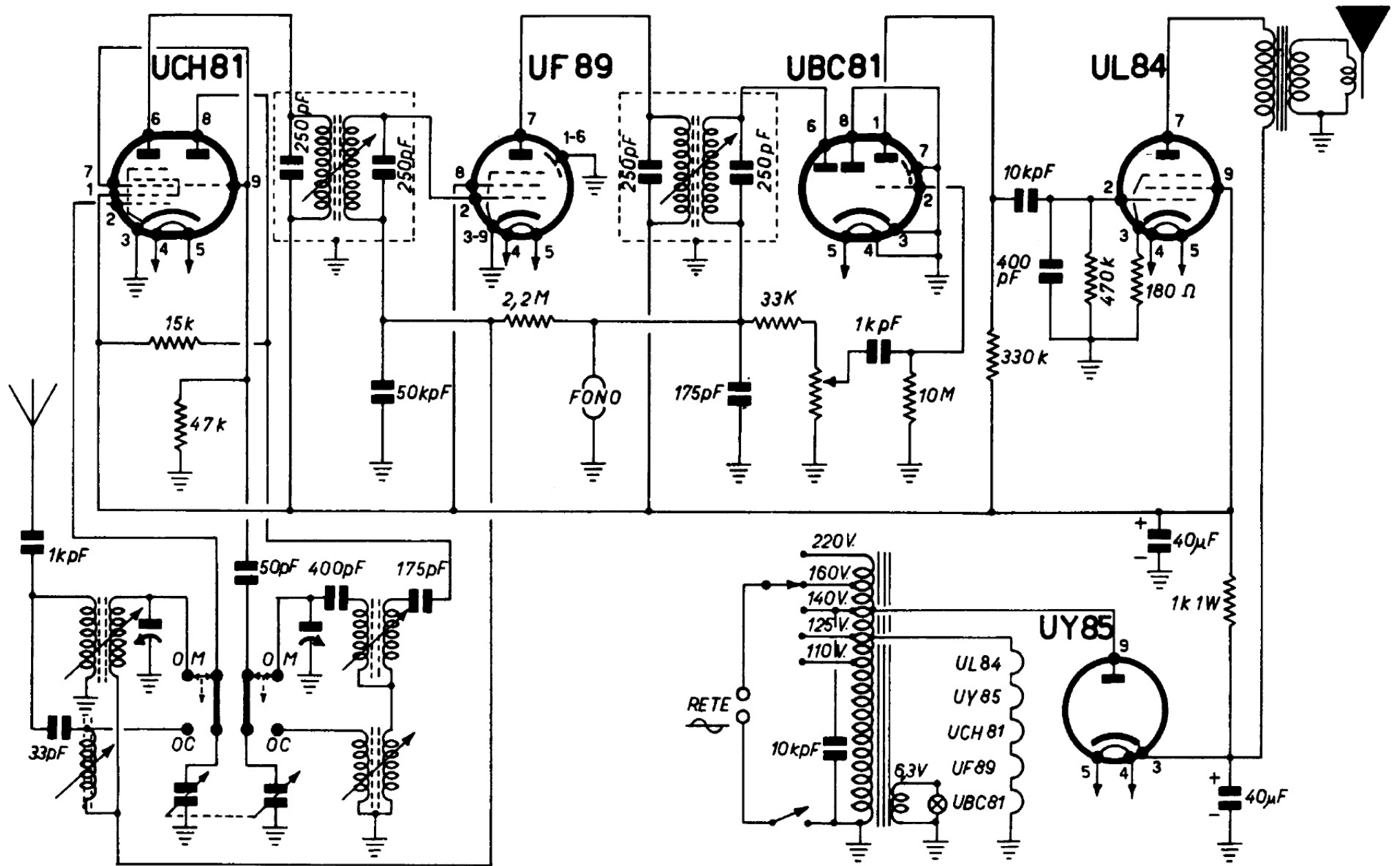
Schema elettrico del radioricevitore OC - OM - Fono AR/3
