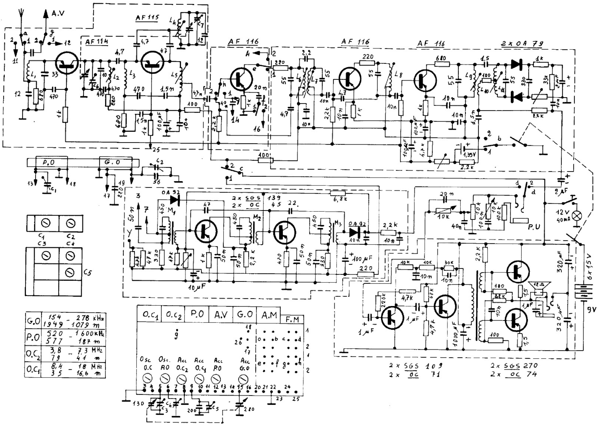
SCHEMA ELETTRICO DEL RADIORICEVITORE G.B.C. AR/50
