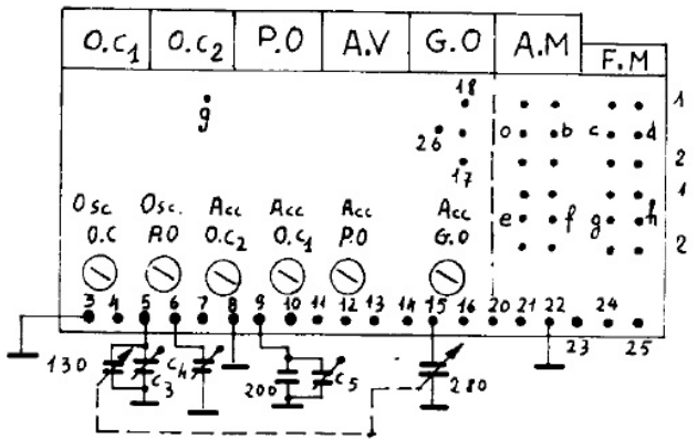
SCHEMA ELETTRICO DEL RADIORICEVITORE G.B.C. AR/50
