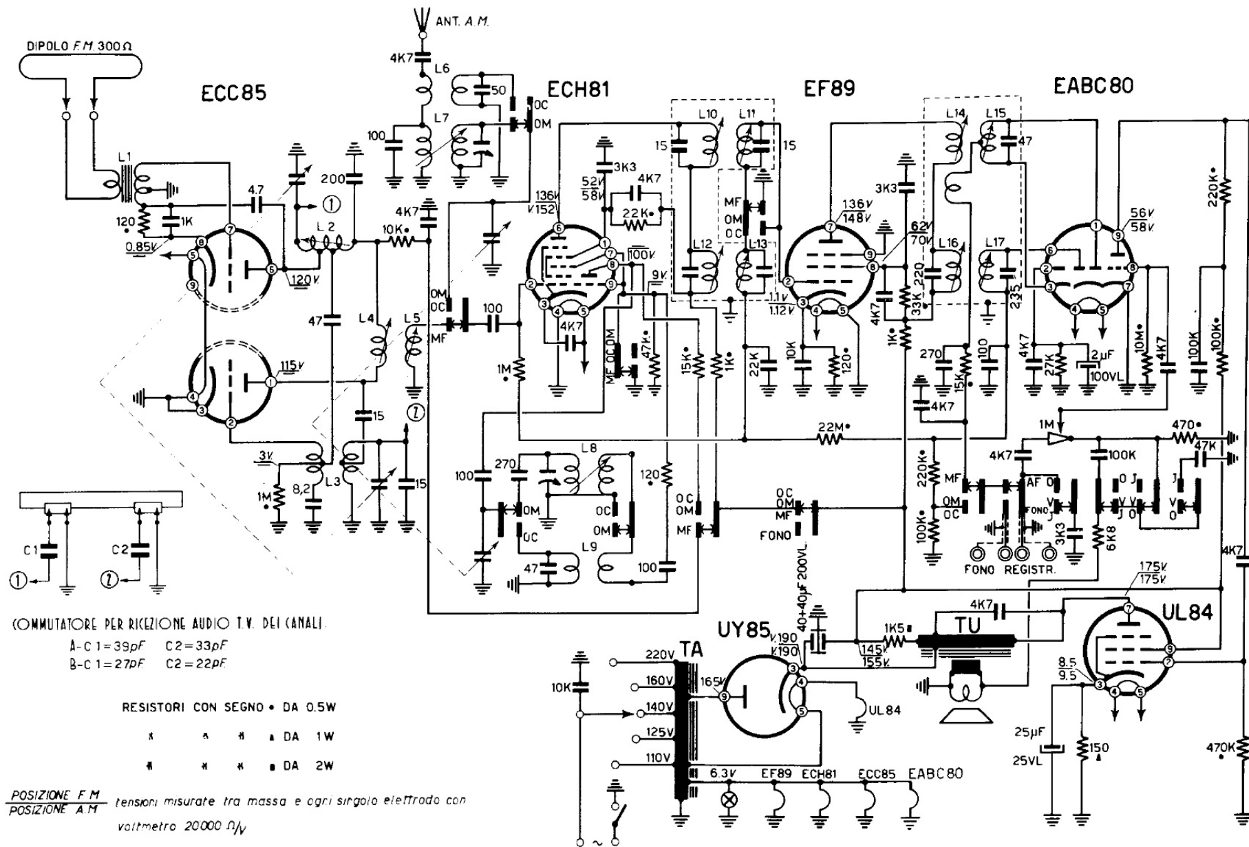
SCHEMA ELETTRICO DEI RADIORICEVITORI G.B.C. FM/4 RECITAL - FM/5 BRIAN - FM/14 CARD E DEI RADIOFONOGRIFI FM/44RF RAMON FM/54RF STARLET - FM/64RF SANGRAU
