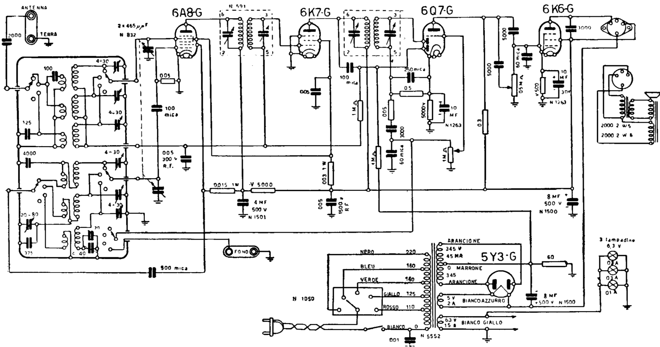
GELOSO. — Mod. G 50R. — Medie, corte e lunghe con AF 1911 A, e medie, corte e cortissime con 1912 A, scala 1776i Media frequenza: 7467 kHz. — Produzione 1935-36.
