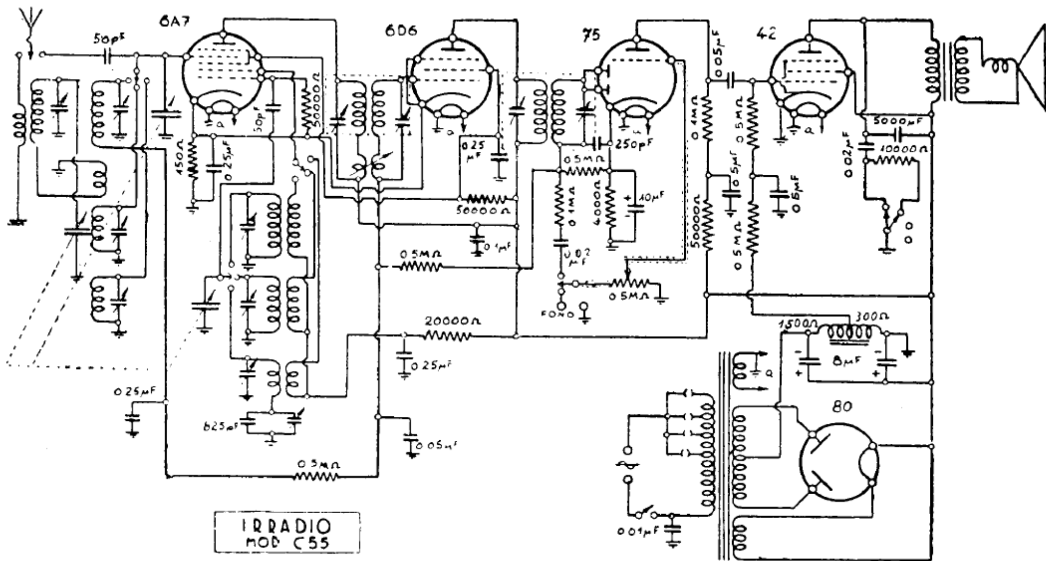
IRRADIO. — Mod. « C 55 ». — Super a 3 gamme d'onda. — Media frequenza: 250 kHz. — Produzione 1937.
