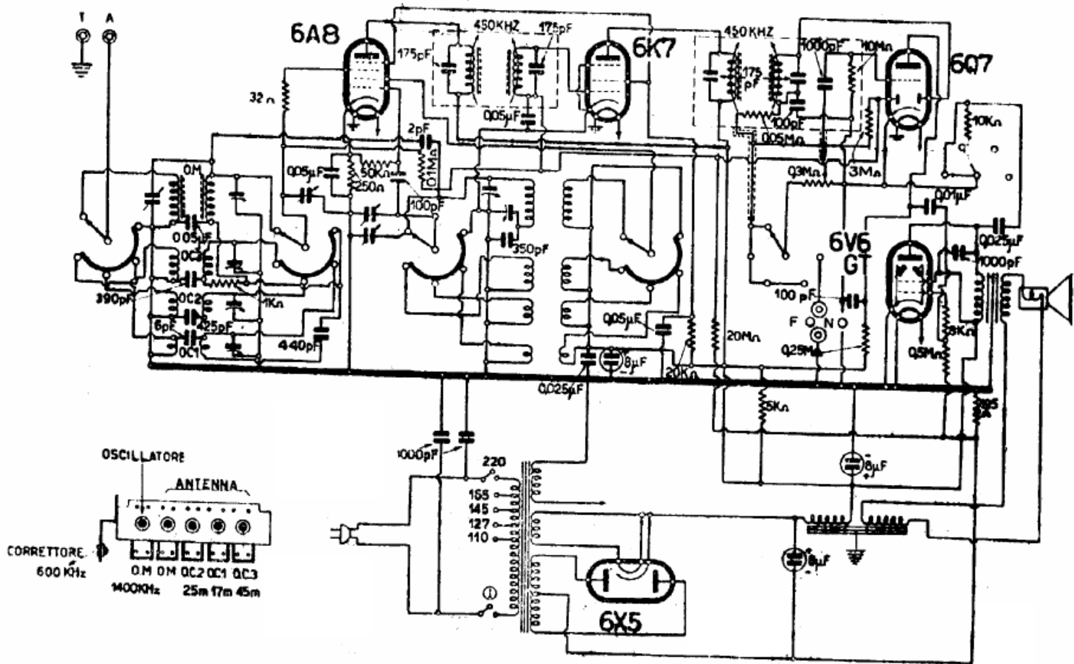
Lo schema elettrico e la posizione dei compensatori del « DL 22 ».
