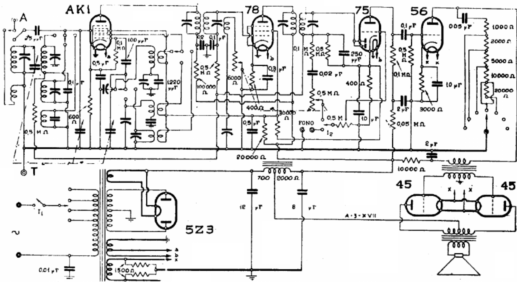
IRRADIO . MOD, « IL RIVELATORE 7 (ALTA FEDELTA') »
