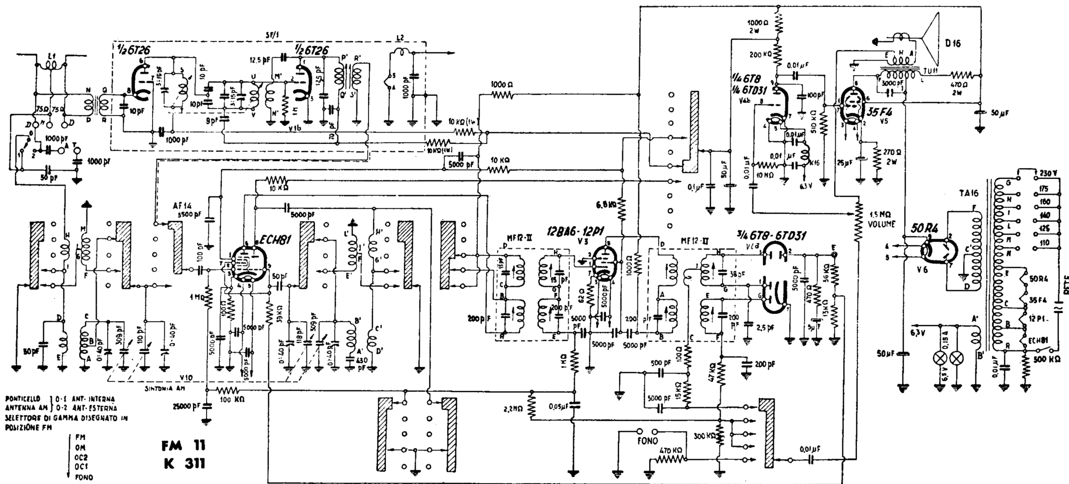
MAGNADYNE RADIO - Modd. FM 11 e K 311. Apparecchio a modulazione d'ampiezza e di frequenza. Onde medie, due gamme onde corte e una banda onde ultracorte a modulazione di frequenza. Media frequenza AM a 471 kc/s, e FM a 10,7 Mc/s. Potenza d'uscita 4 watt.
