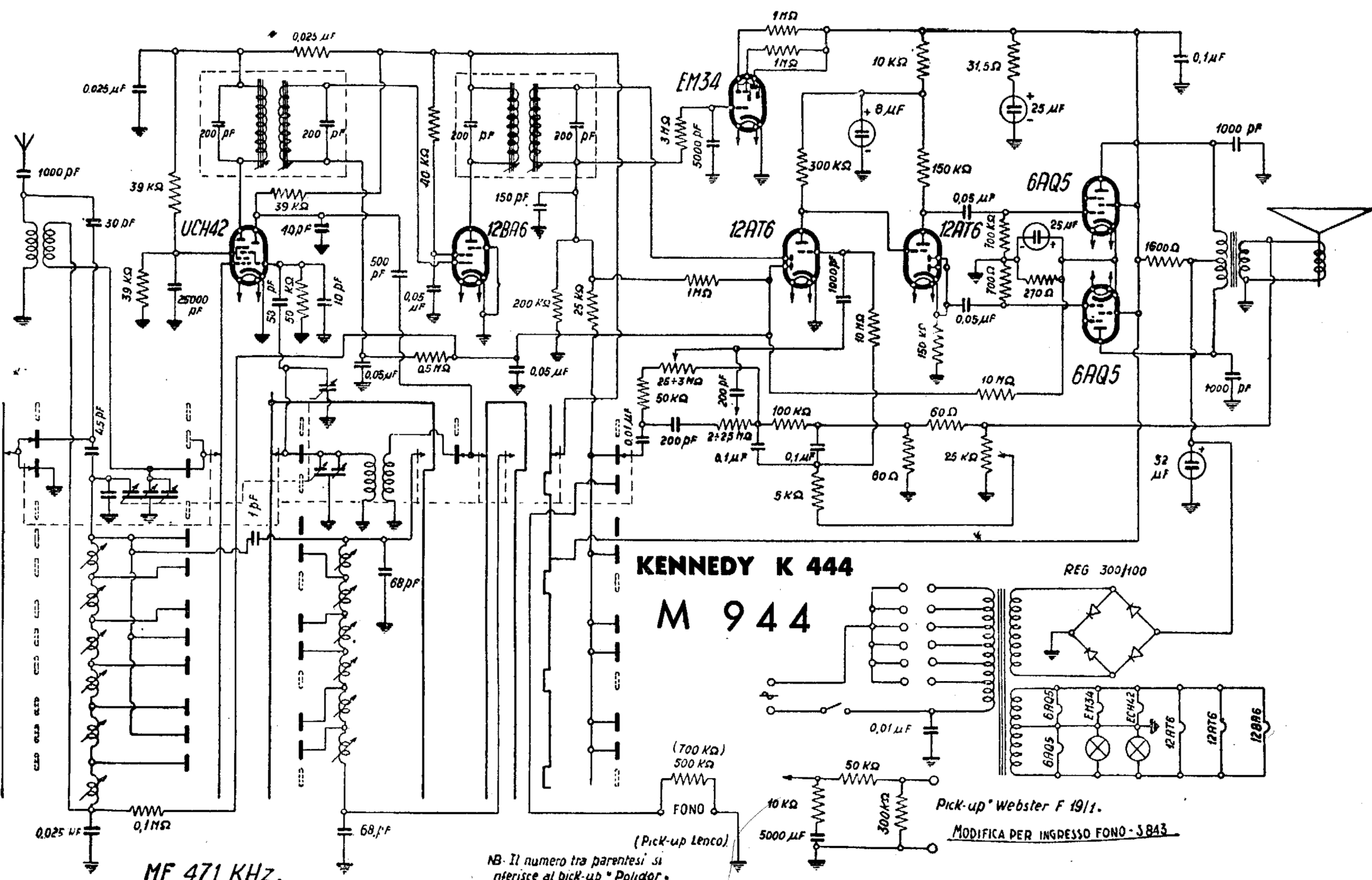
MAGNADYNE RADIO - Modd. KENNEDY K 444 e DAMAITER M 944. Una gamma onde medie e sei bande allargate onde corte e cortissime. Media frequenza 471 kc/s. Controllo volume con compensazione toni bassi. Potenza indistorta di uscita 10 watt.
