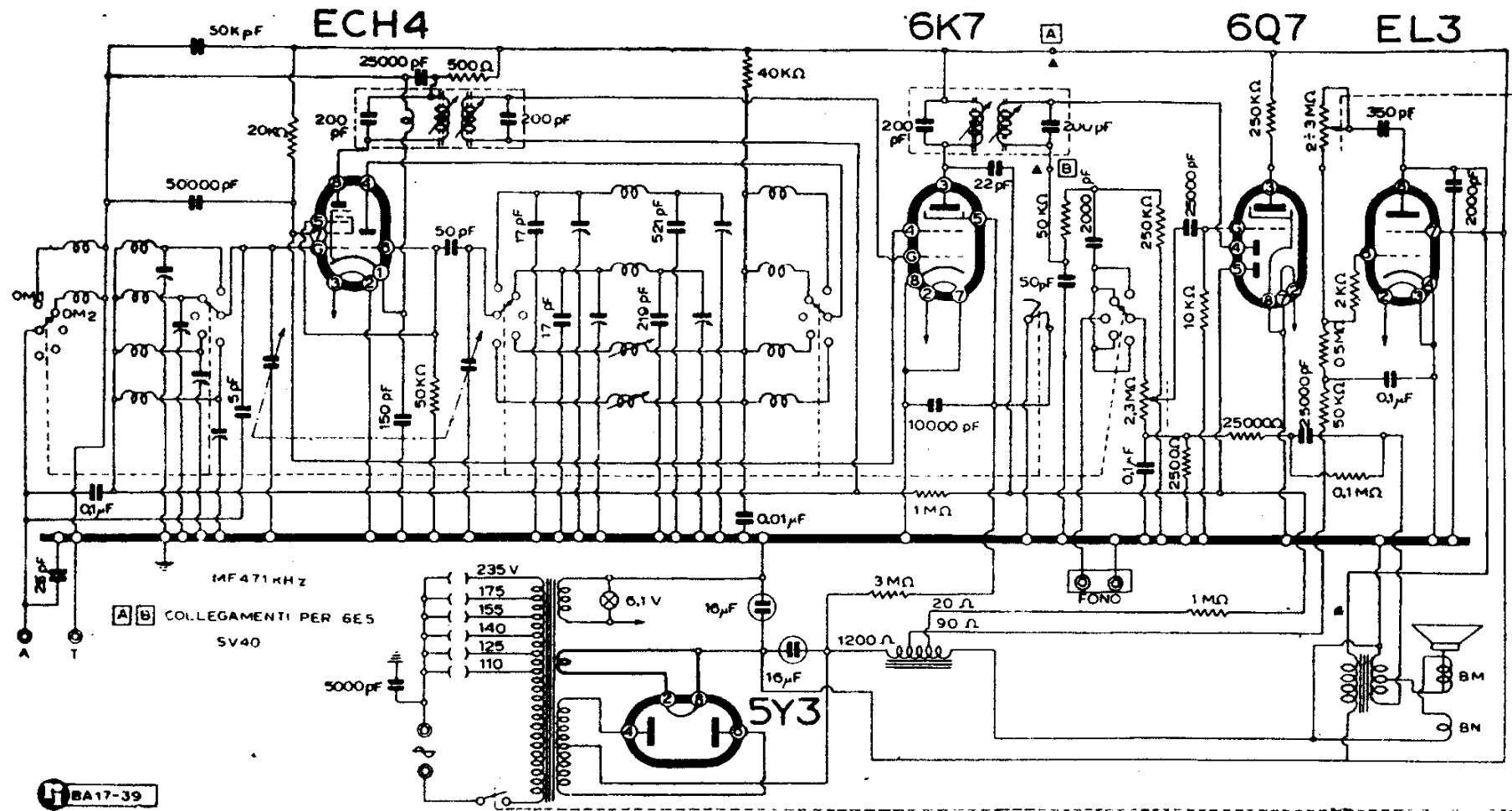
MAGNADYNE - MOD. « SV 37 »
