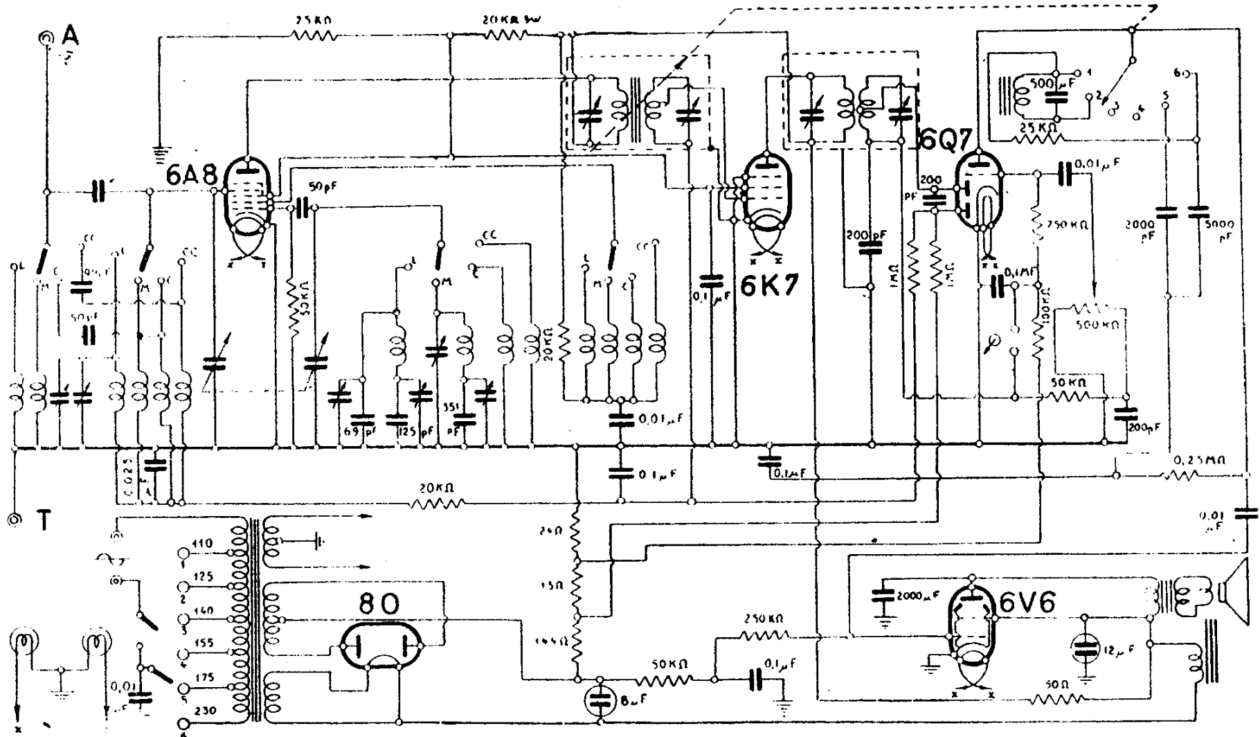
MAGNADYNE - MODD. « SV 56 » « SV 56 C »
