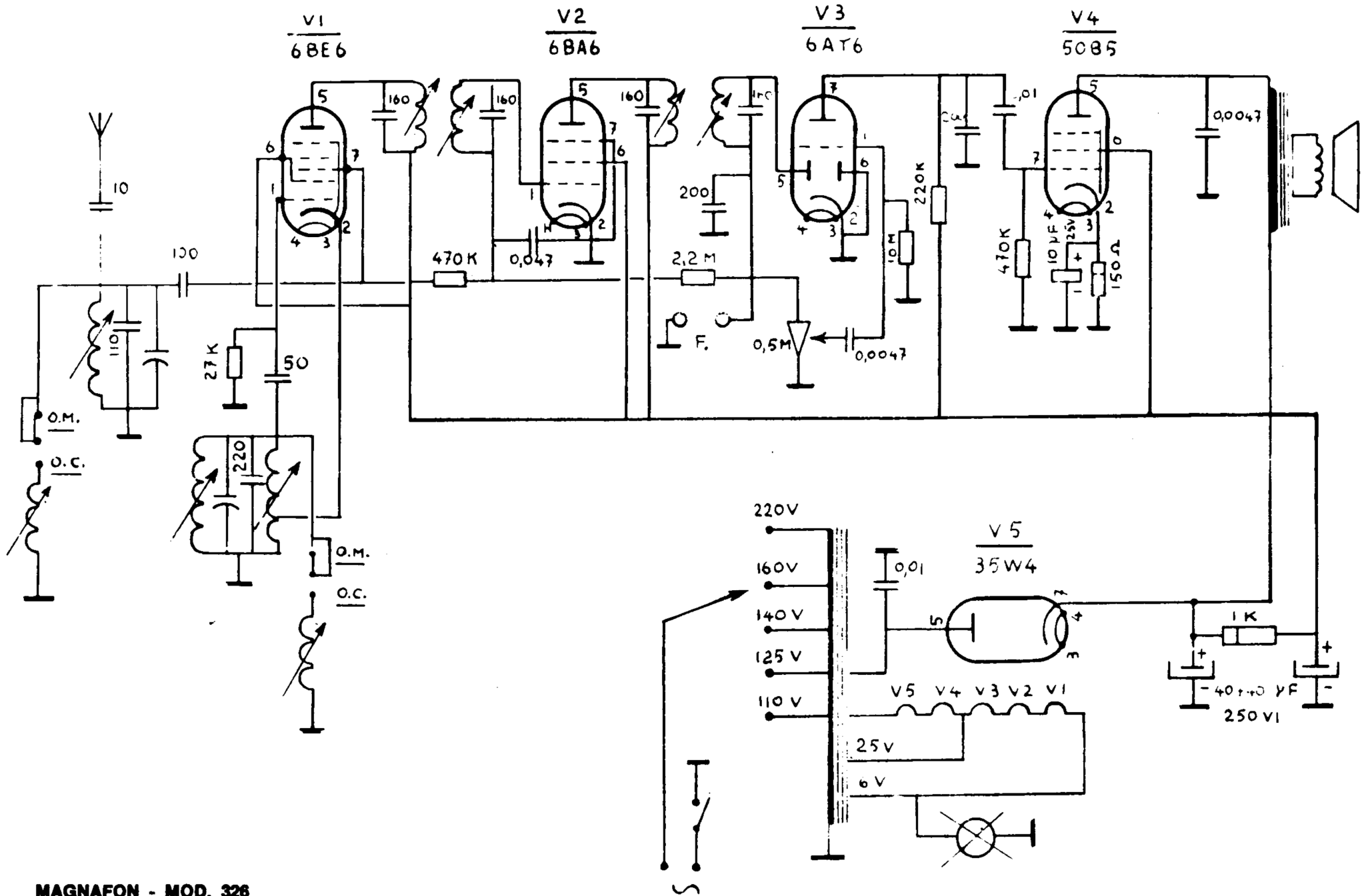
MAGNAFON - MOD. 326
