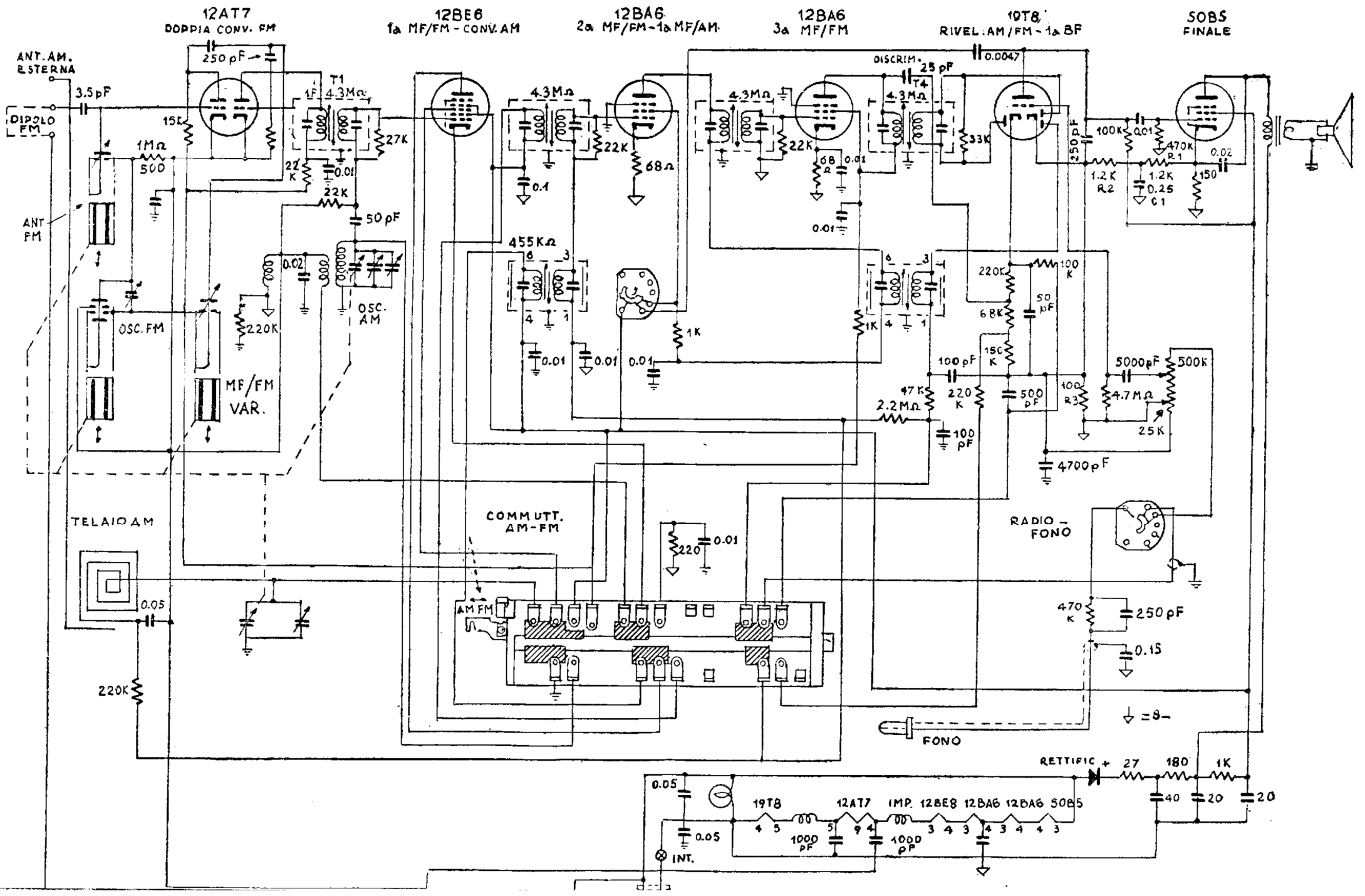
Fig. 15.9. - Supereterodina AM-FM, con circuiti accordati a cavo coassiale e doppia conversione di frequenza. (Motorola mod. 77FM21).
