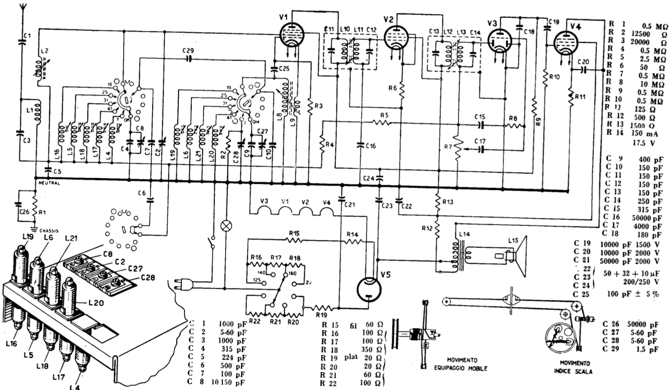
RADIO MARELLI - Mod. 131 B. Onde medie da 518 a 1610 kc/s; onde tropicali da 2800 a 6500 kc/s; banda 41 m da 7000 a 7500 kc/s; banda 31 m da 9465 a 9870 kc/s; banda 25 m da 11.639 a 12.000 kc/s; banda 19 m da 15.025 a 15.400 kc/s. Media frequenza 455 kc/s. Valvole: V1 - 12BE6; V2 - 12BA6; V3 - 12AT6; V4 - 35QL6; V5 - 35X4.
