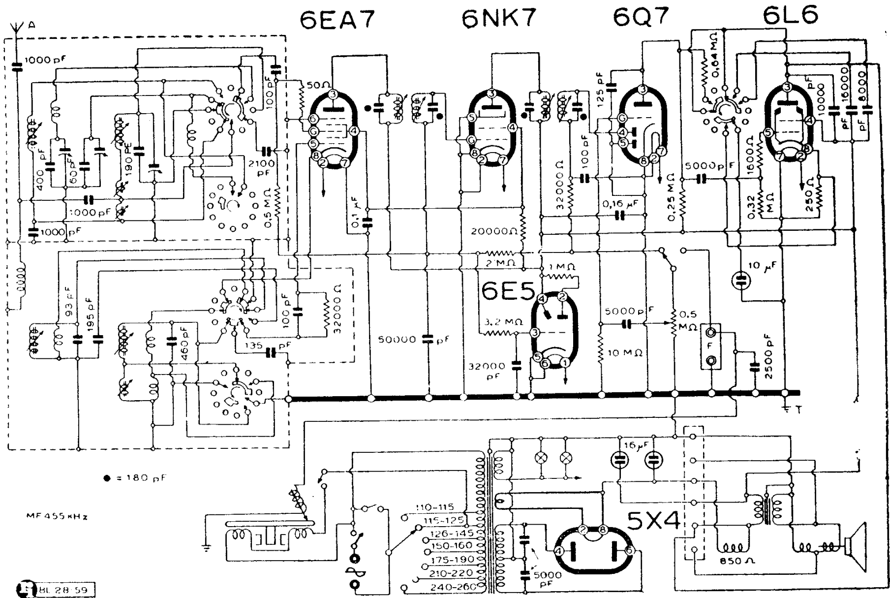
RADIOMARELLI - MOD. « 9F95 »
