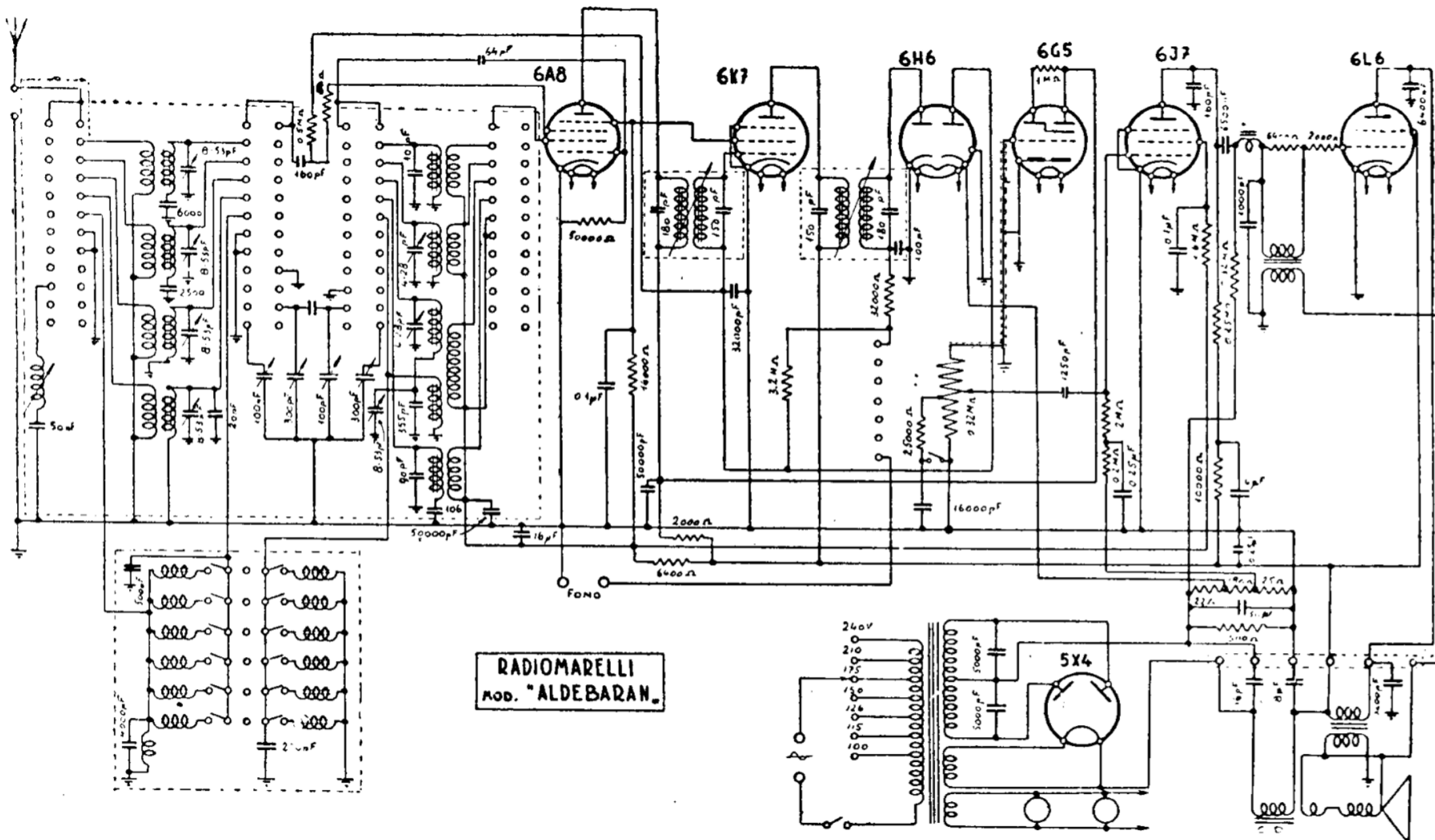
RADIO MARELLI. — Modelli Aldebaran e Aldebaran fono. — Produzione 1938-39. — Gamme: cc. (19-30), c. (30-50), m. (200-570), l. (1000-2000). — Potenza d'uscita 5,5 W. — Media frequenza: 450 kHz.
