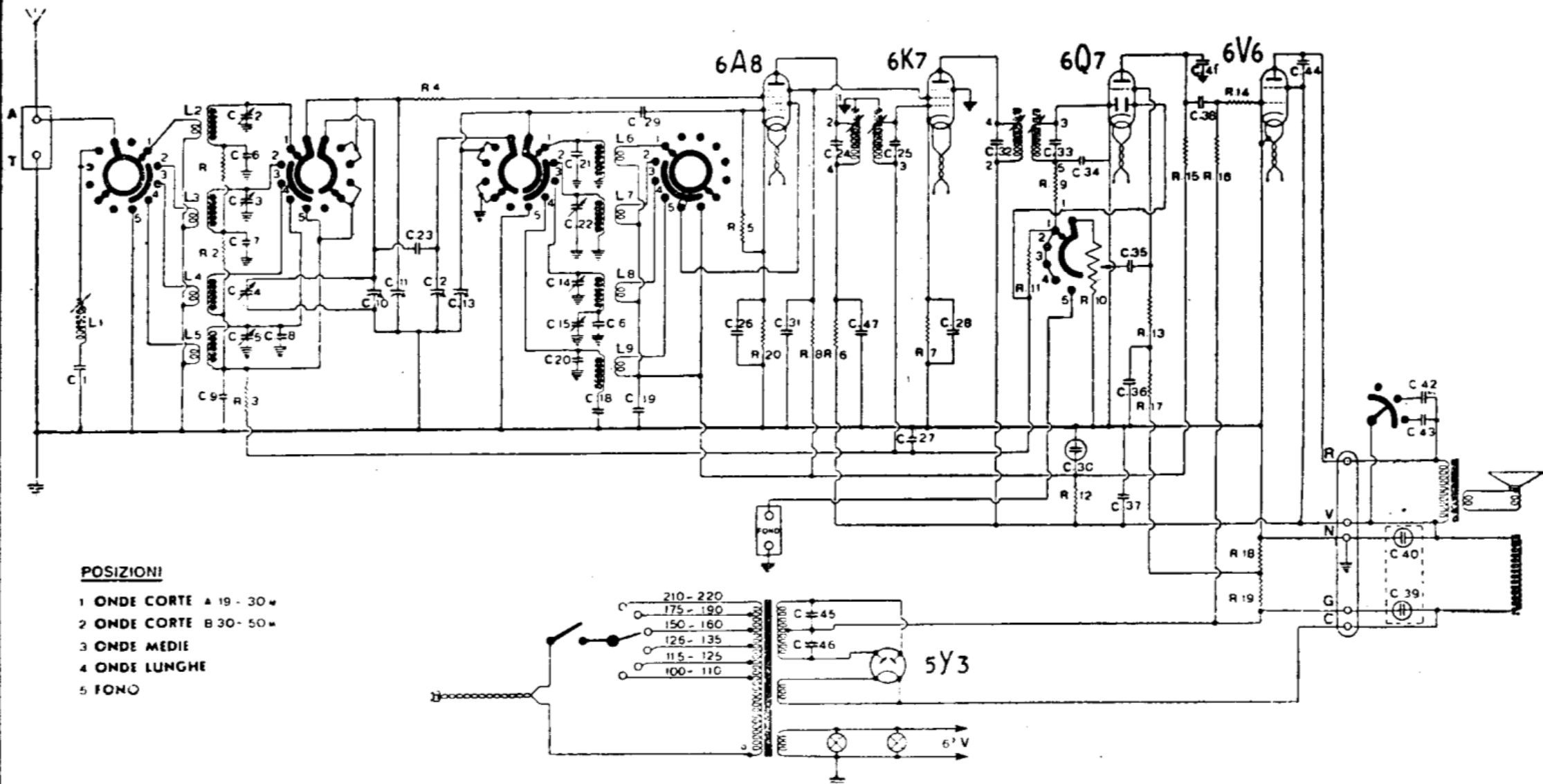
Fig. 182. — RADIO MARELLI. - Mod. «ALTAIR». Schema elettrico per la taratura di cui le norme a pag. 275. Per valori dei condensatori e resistenze vedi «Radio Libro», V ediz., pag. 367.
