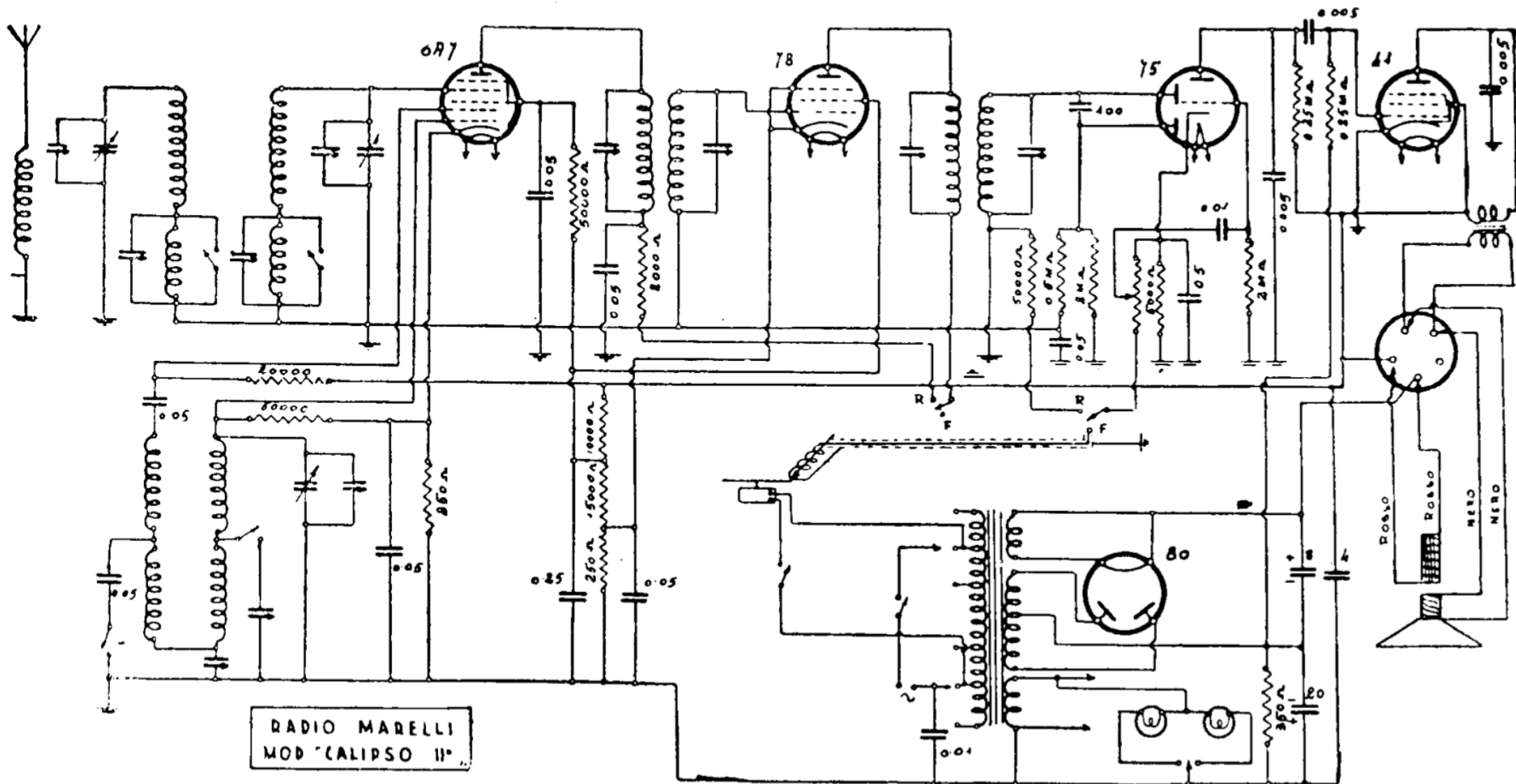
RADIO MARELLI. — « Modelli Calipso II e Damayante ». Anno di produzione 1394. — Media frequenza: 125 kc. (Il secondo condensatore variabile non va collegato di circuito c.a.v. come indicato; va solo a massa; il circuito di placca della 78 va collegato al massimo anodica).
