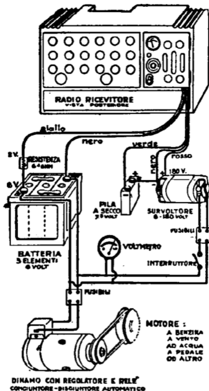
L'impianto di manutenzione del radiorecettore coloniale « Dubat » con batteria e survoltore.
