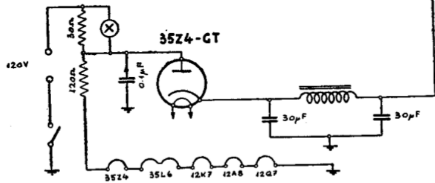
Fig. 10.4. - Ricevitore « FIDO » (Radio Marelli), adatto per alimentazione sia con corrente alternata che continua., sprovvisto di trasformatore di alimentazione.
