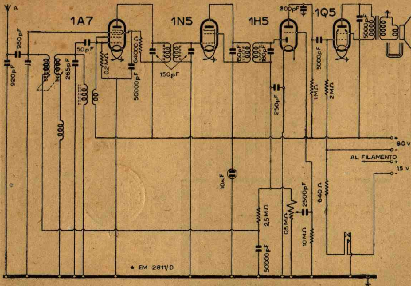
Lo schema elettrico del Fido a pile
