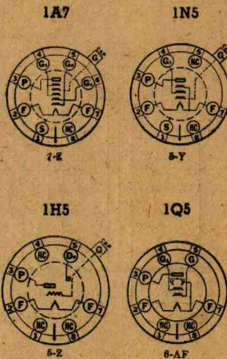
Le valvole del Fido a pile
