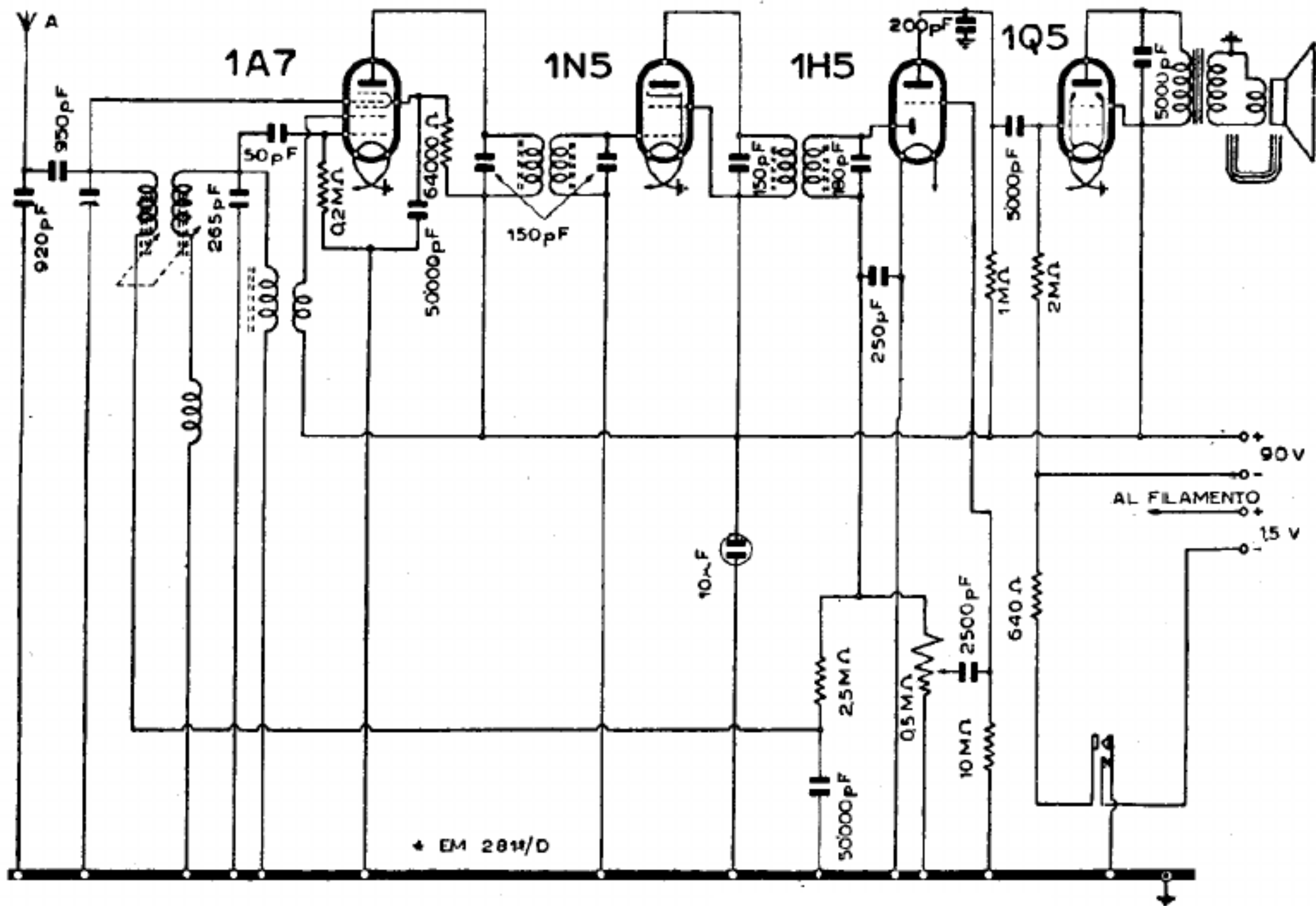
RADIOMARELLI - MOD. « FIDO A PILE »
