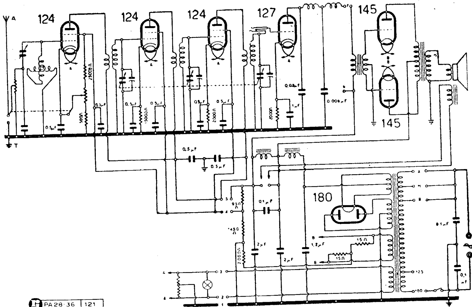
RADIOMARELLI - MOD. « MUSAGETE I »
