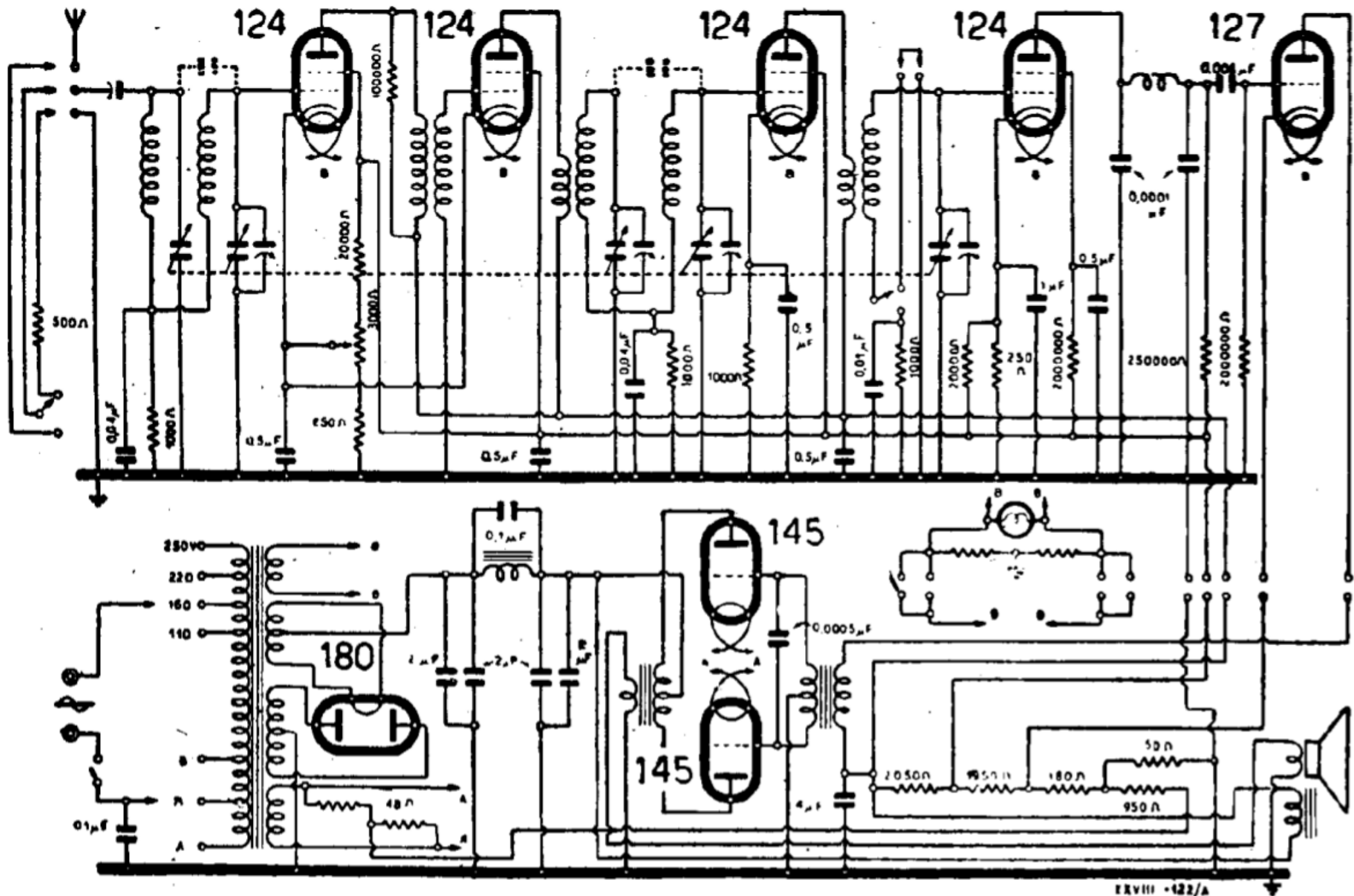
RADIOMARELLI - MOD. «MUSAGETE II»
