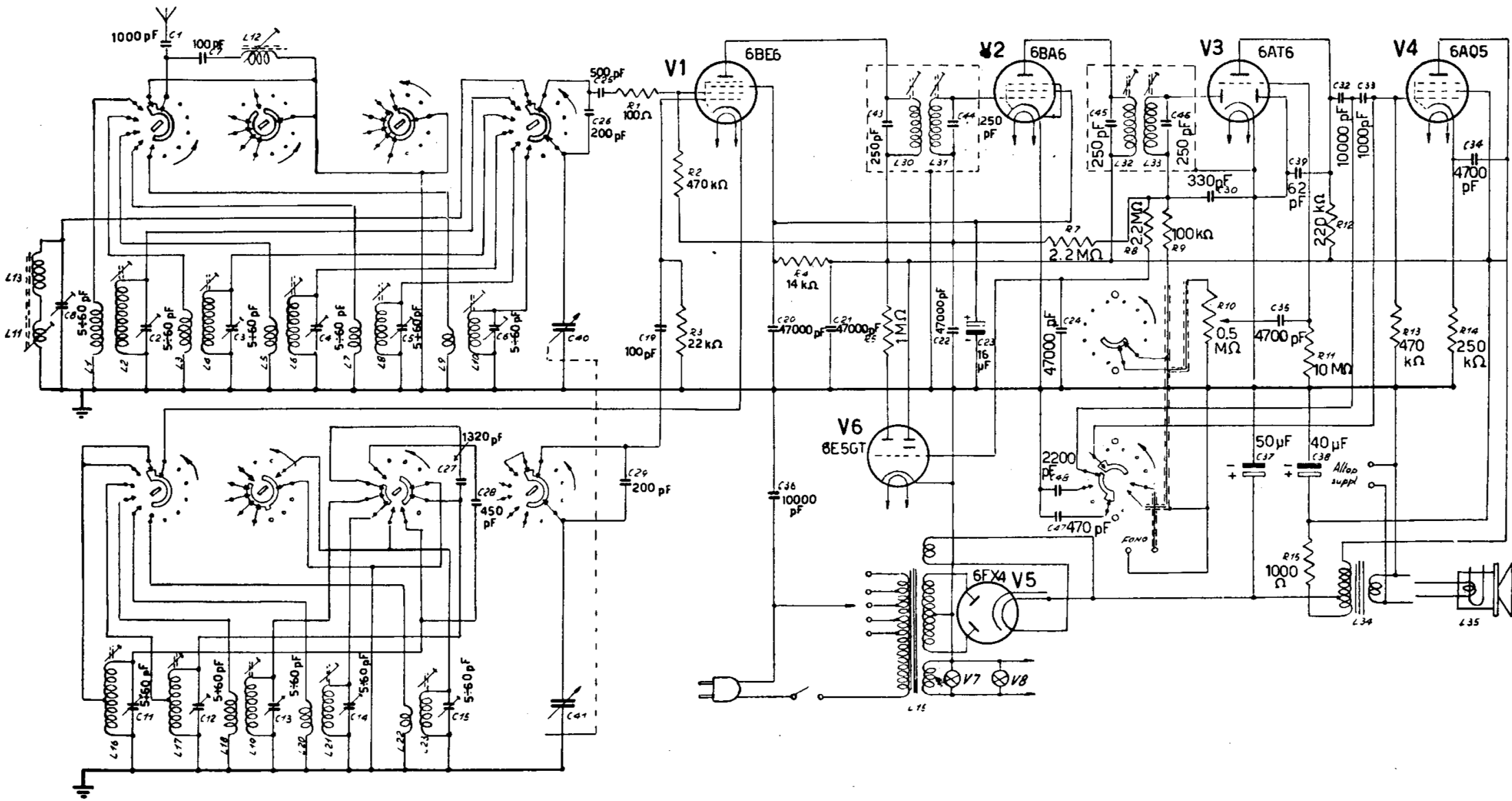
RADIO MARELLI - Mod. RD147. Una gamma onde medie; una gamma onde medie-corte (tropicali) e tre bande allargate onde corte. Media frequenza 455 kc/s.
