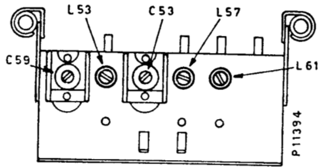
Gruppo R.F. Mod. di amp. - Vista posteriore
