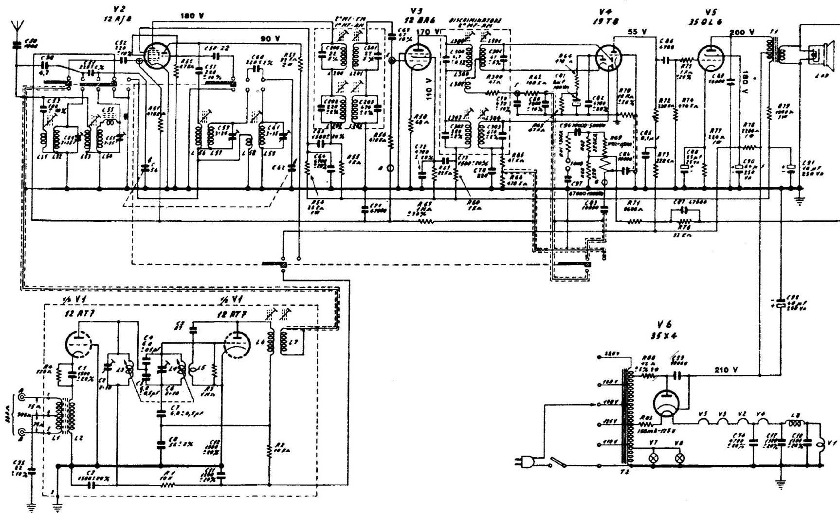
RADIOMARELLI - MODD. RD180MF - RD206MF - RD213MF
