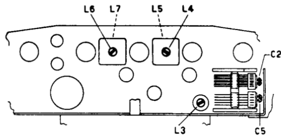
CONDENSATORI E INDUTTANZE REGOLABILI
