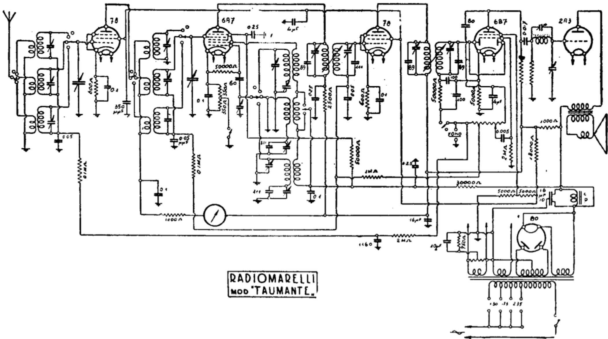
RADIO MARELLI. — Modello « Taumante ». - Produzione 1935 - Media frequenza: 456 kc.
