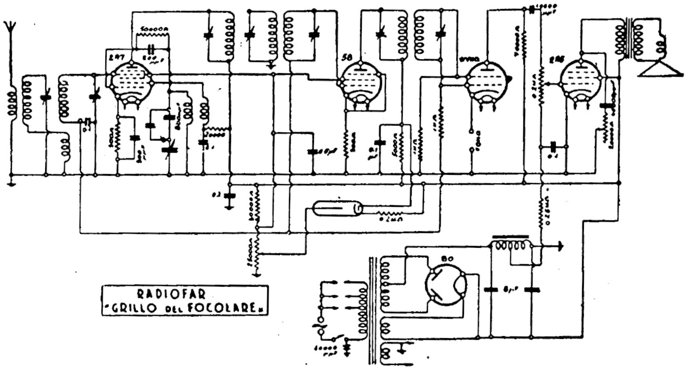
S. A. RADIOFAR. — Modello « Grillo del Focolare ». - Produzione 1934. - Media frequenza: 175 kc.
