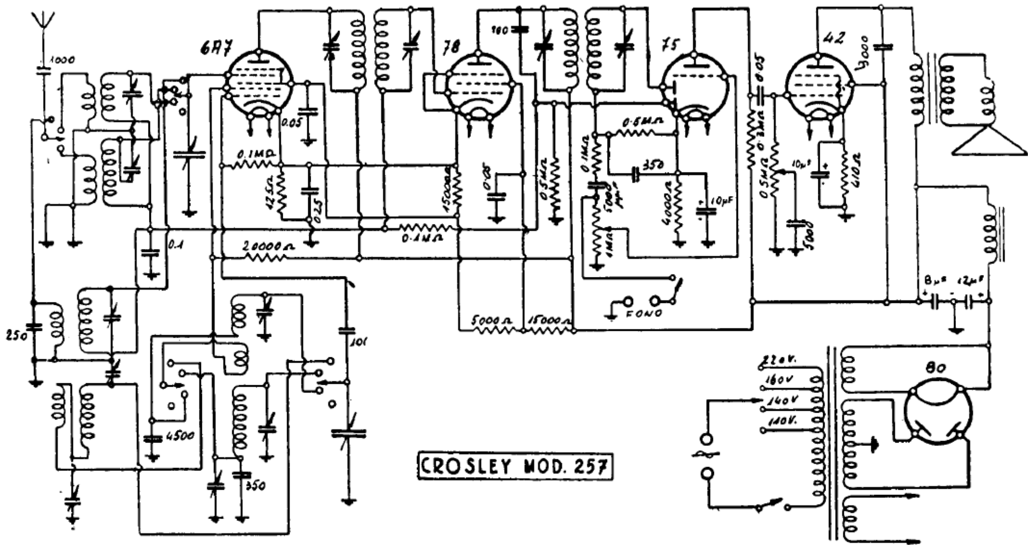
CROSLY RADIO. — Modello « 257 A ». • Produzione 1935. • Media frequenza: 348. kc
