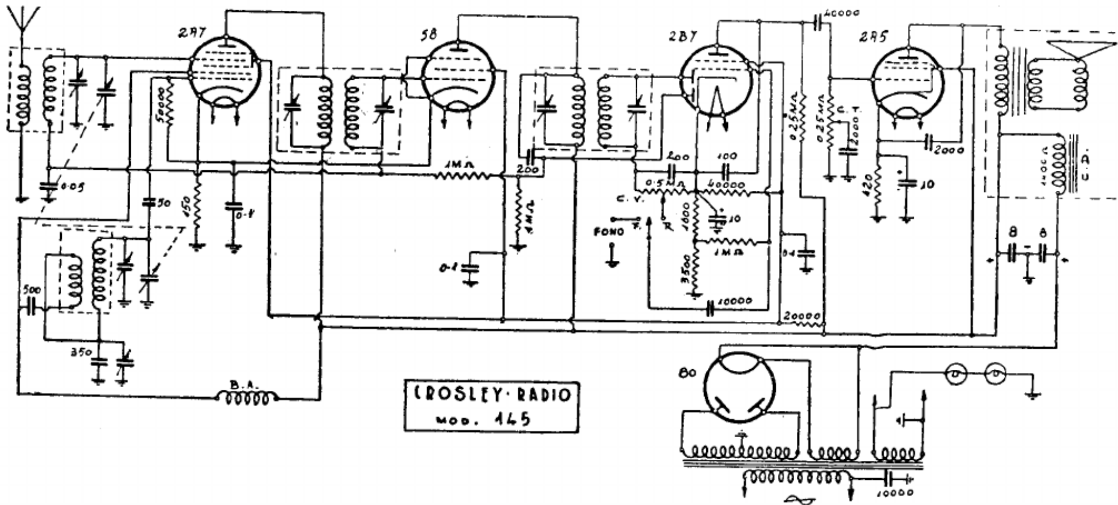
CROSLEY RADIO. — Modello « 145 ». - Produzione 1934. - Media frequenza: 350 kc.
