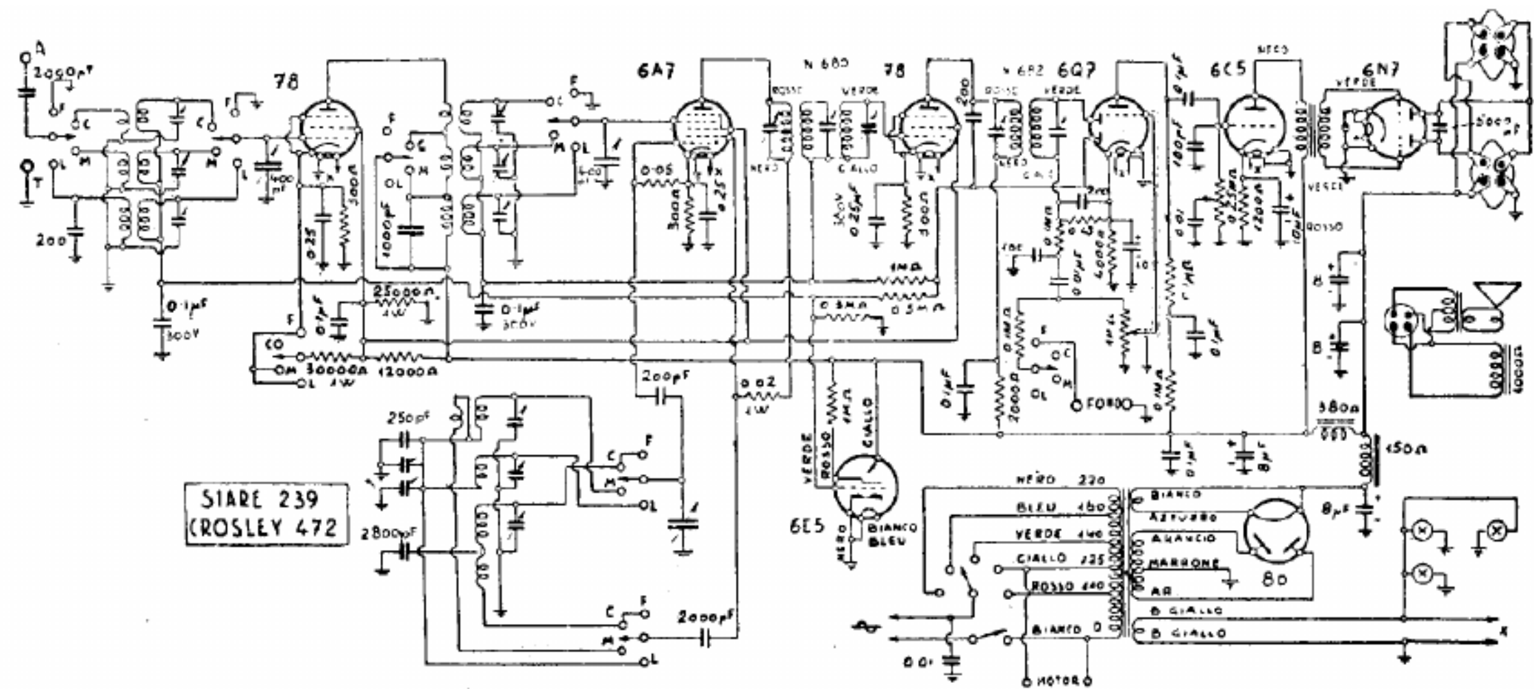
RADIO SIARE. — Modelli « Siare 239 » e « Crosley 472 » a onde corte medie e lunghe; con sintonizzatore visivo a tubo a raggi catodici (6E5). - Produzione 1937. - Media frequenza: 468 kHz.
