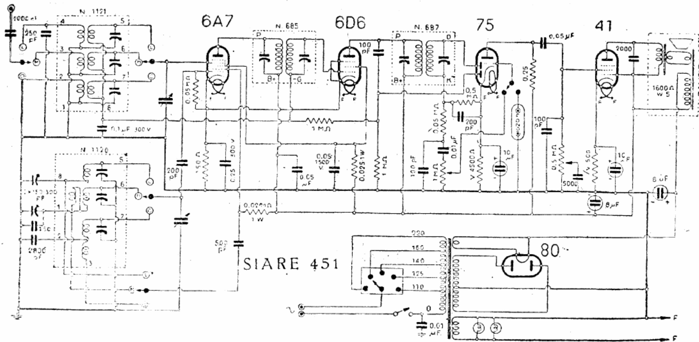
RADIO SIARE. — Mod. 451. — Produzione 1938-39. — Potenza d'uscita: 8 W. — Media frequenza: 467 kHz.
