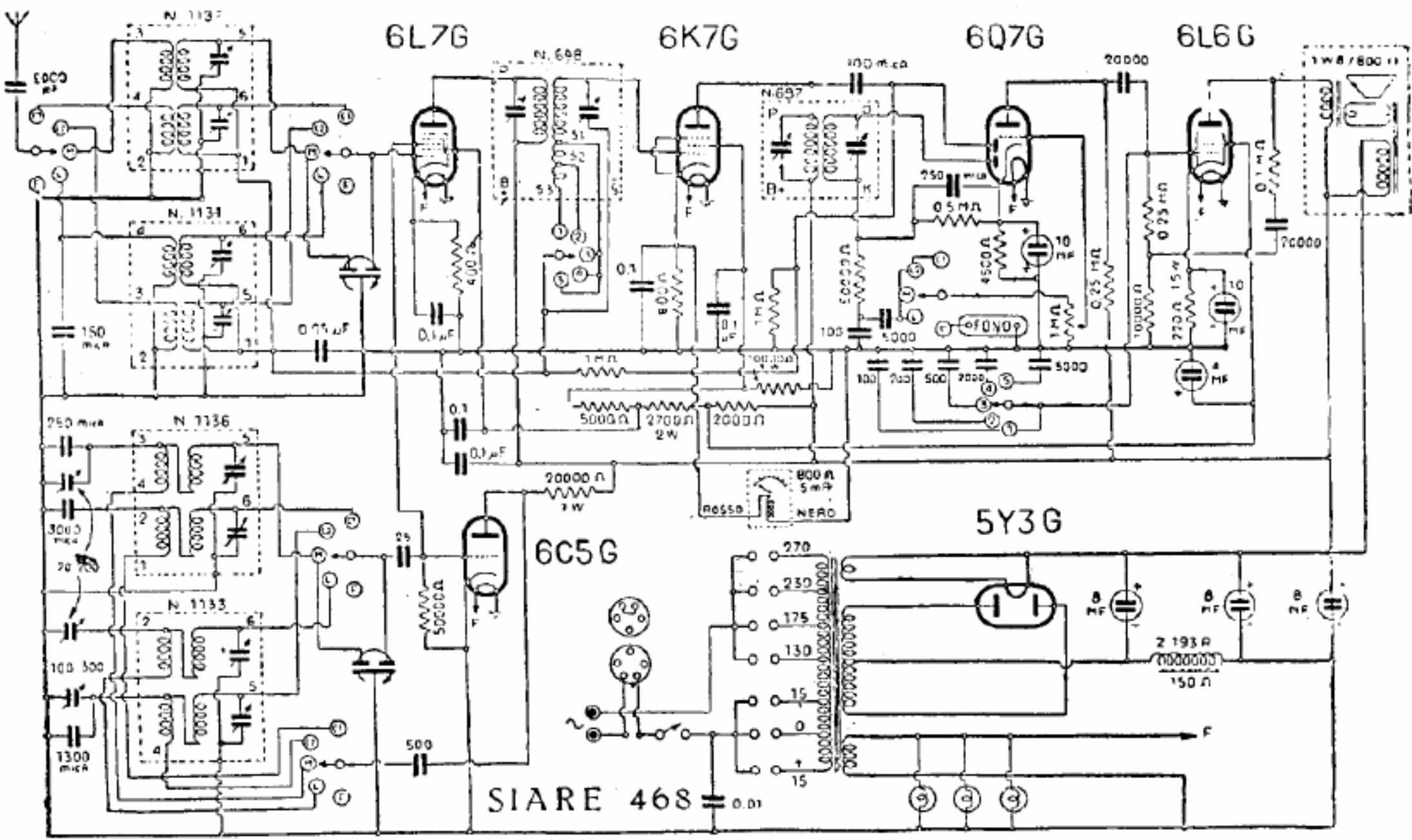
RADIO SIARE. — Mod. 468. — Produzione 1938-39. — Media frequenza: 467 kHz.
