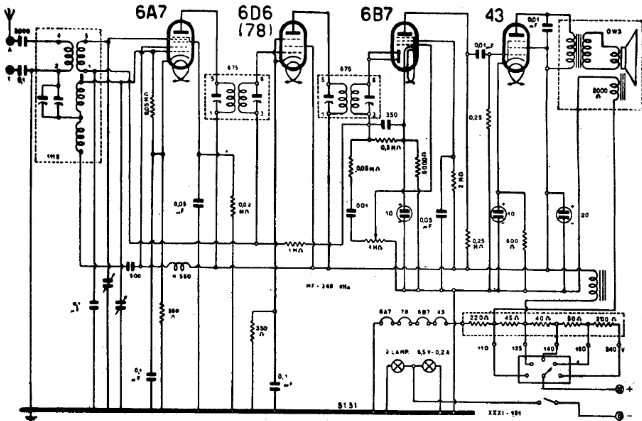
S.I.A.R.E. CROSLY - MOD. « 7411 D. C. »
