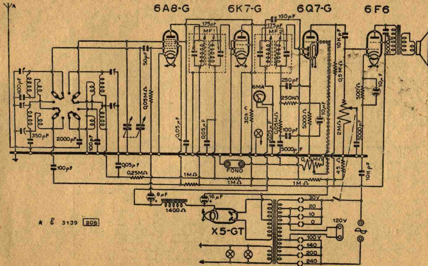
Lo schema elettrico del mod. "501,, Siare (telato 2521).
