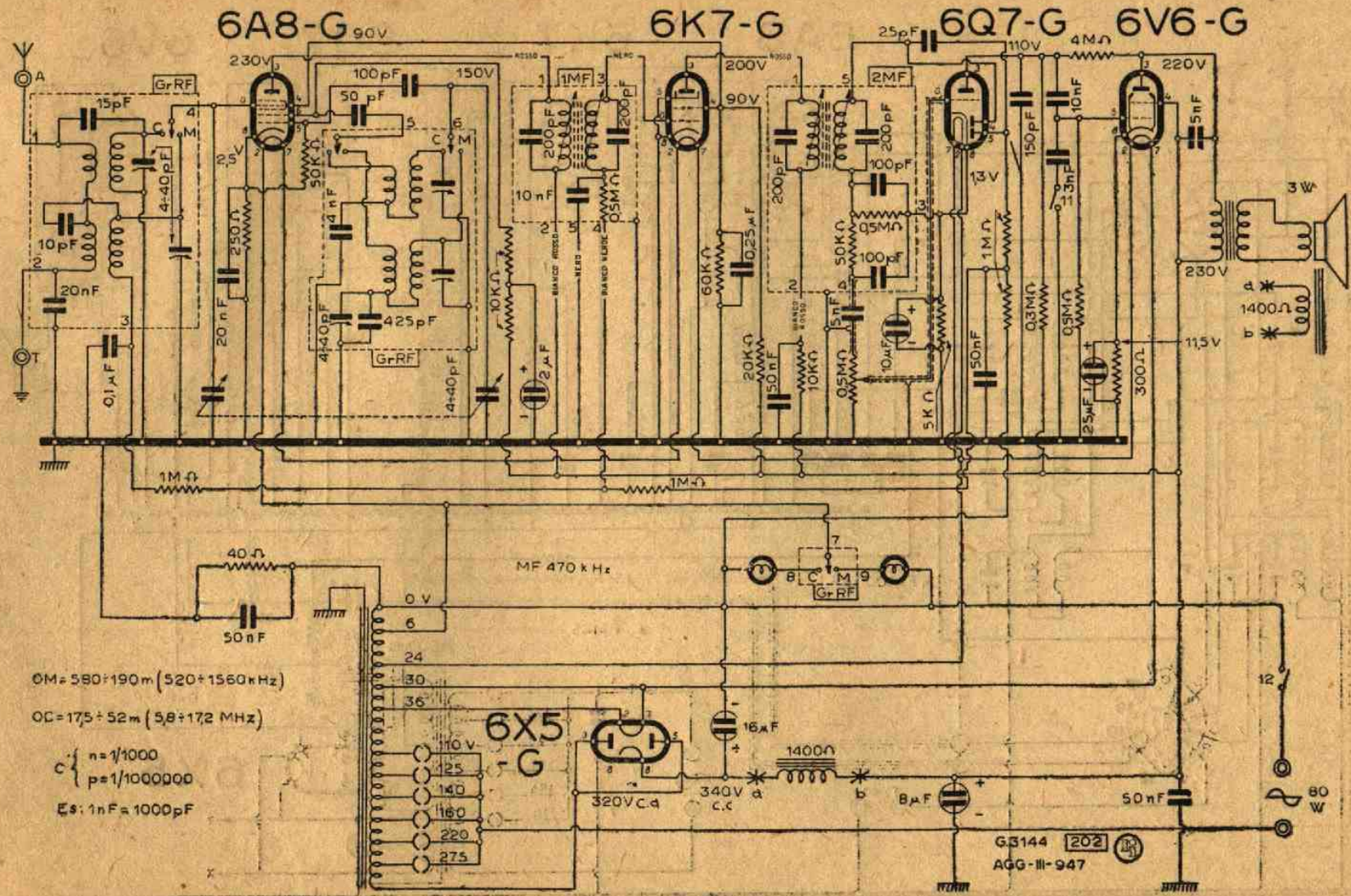
Lo schema elettrico del mod. RR 11 Siare.
