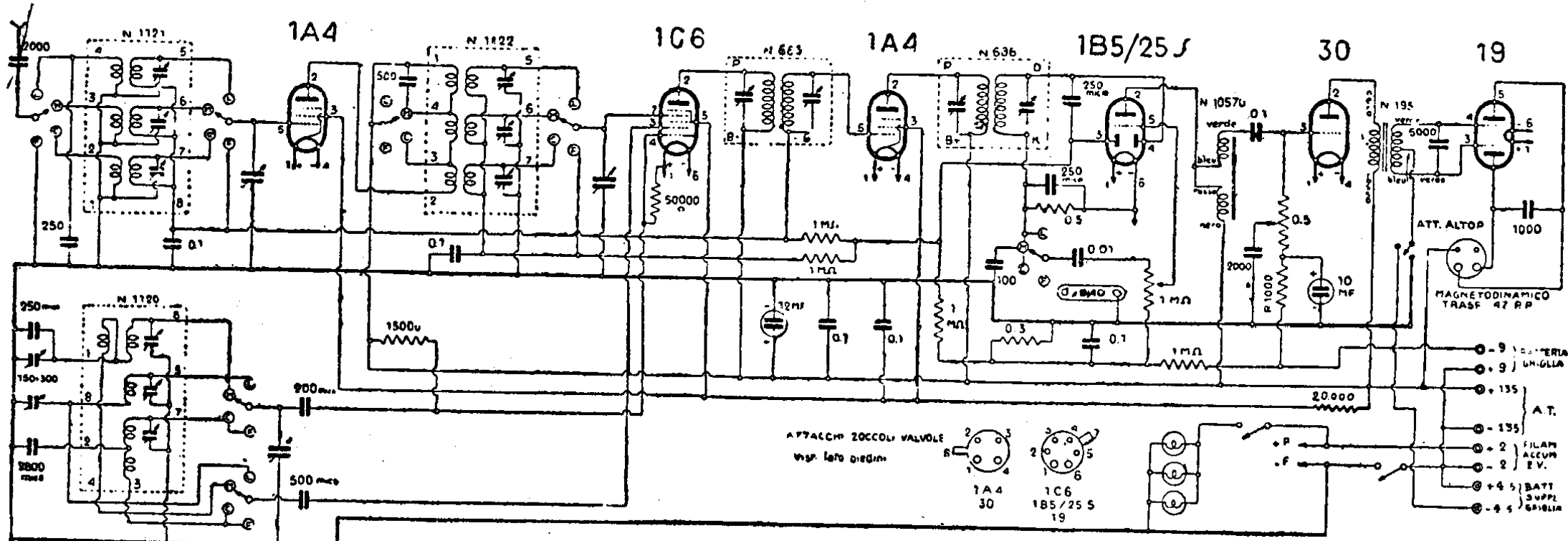
SCHEMA ELETTRICO 8632 SIARE 414-E
