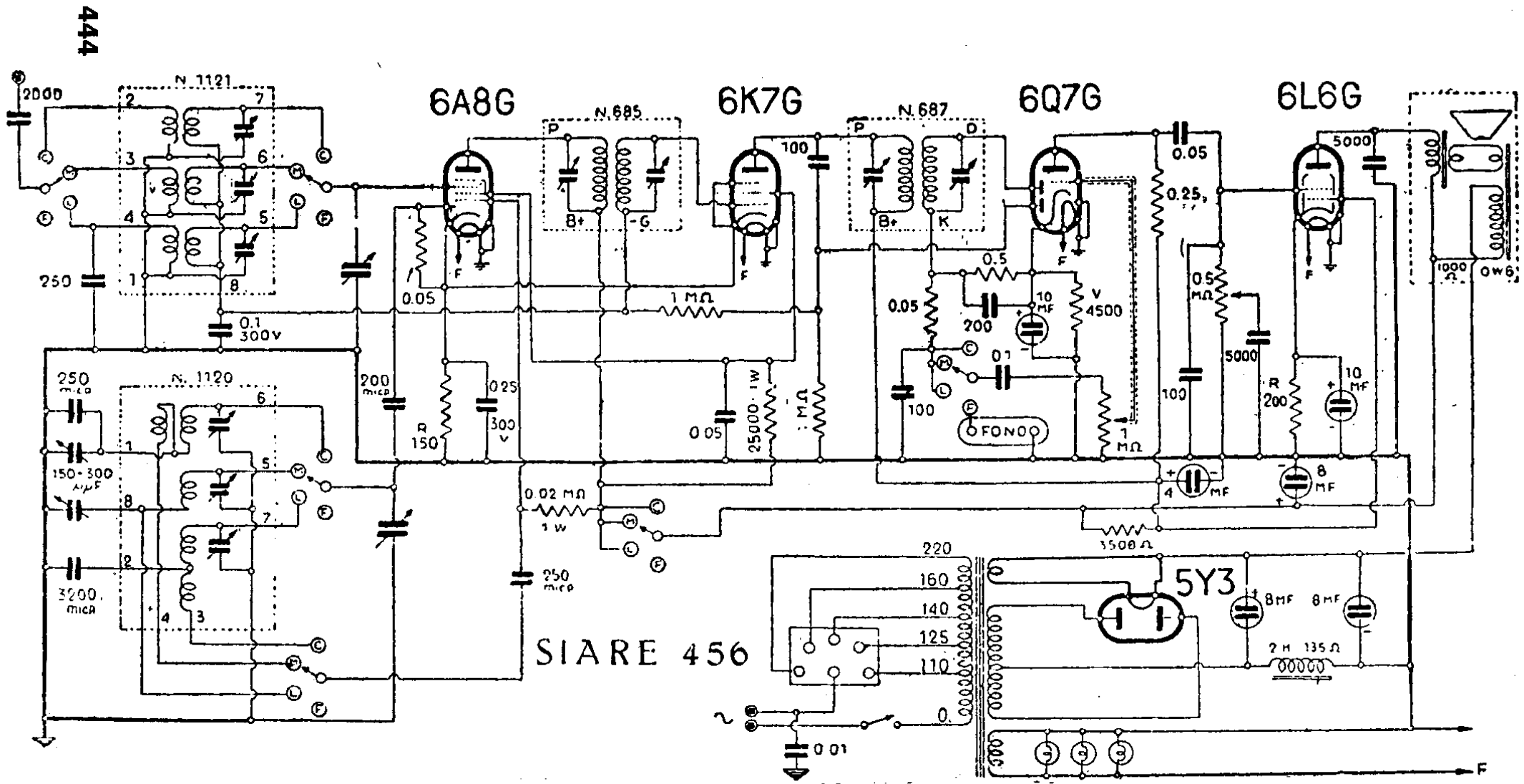
RADIO SIARE. — Mod. « 456 » e « Crosley 255 ». — Produzione 1938-39. — Media frequenza: 467 kHz.
