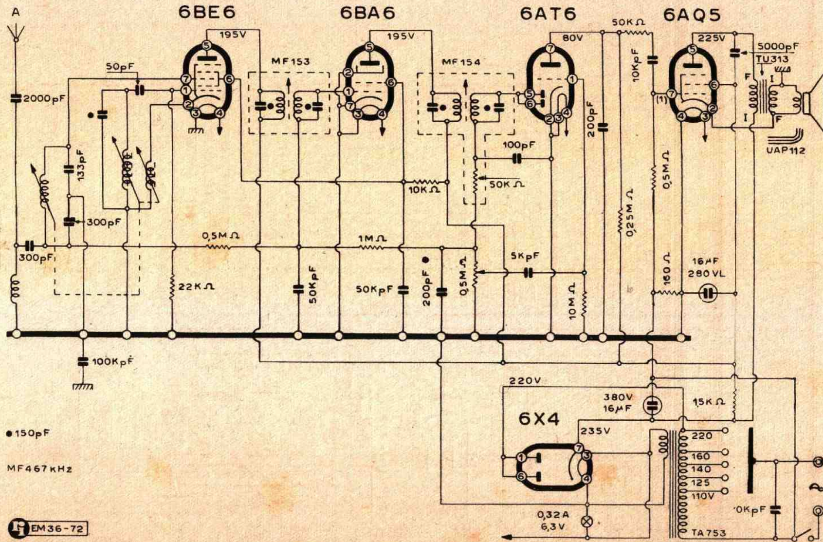
Lo schema elettrico del mod. Mono Unda 51/2
