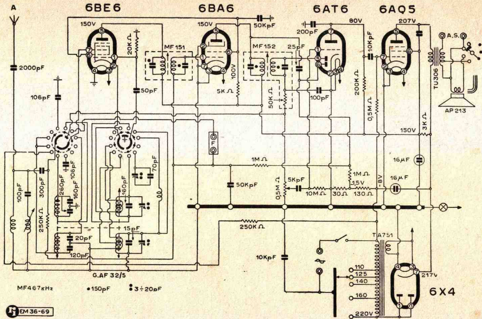
Lo schema elettrico del mod. Tri-Unda 53/18 Undina
