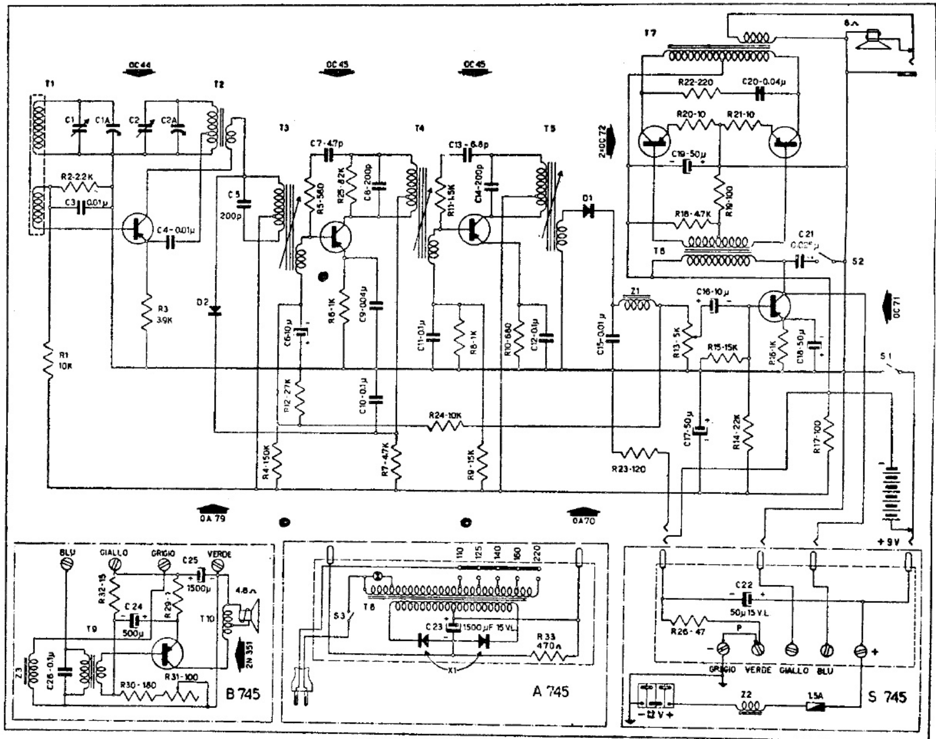
SCHEMA ELETTRICO 745. 1-5513
