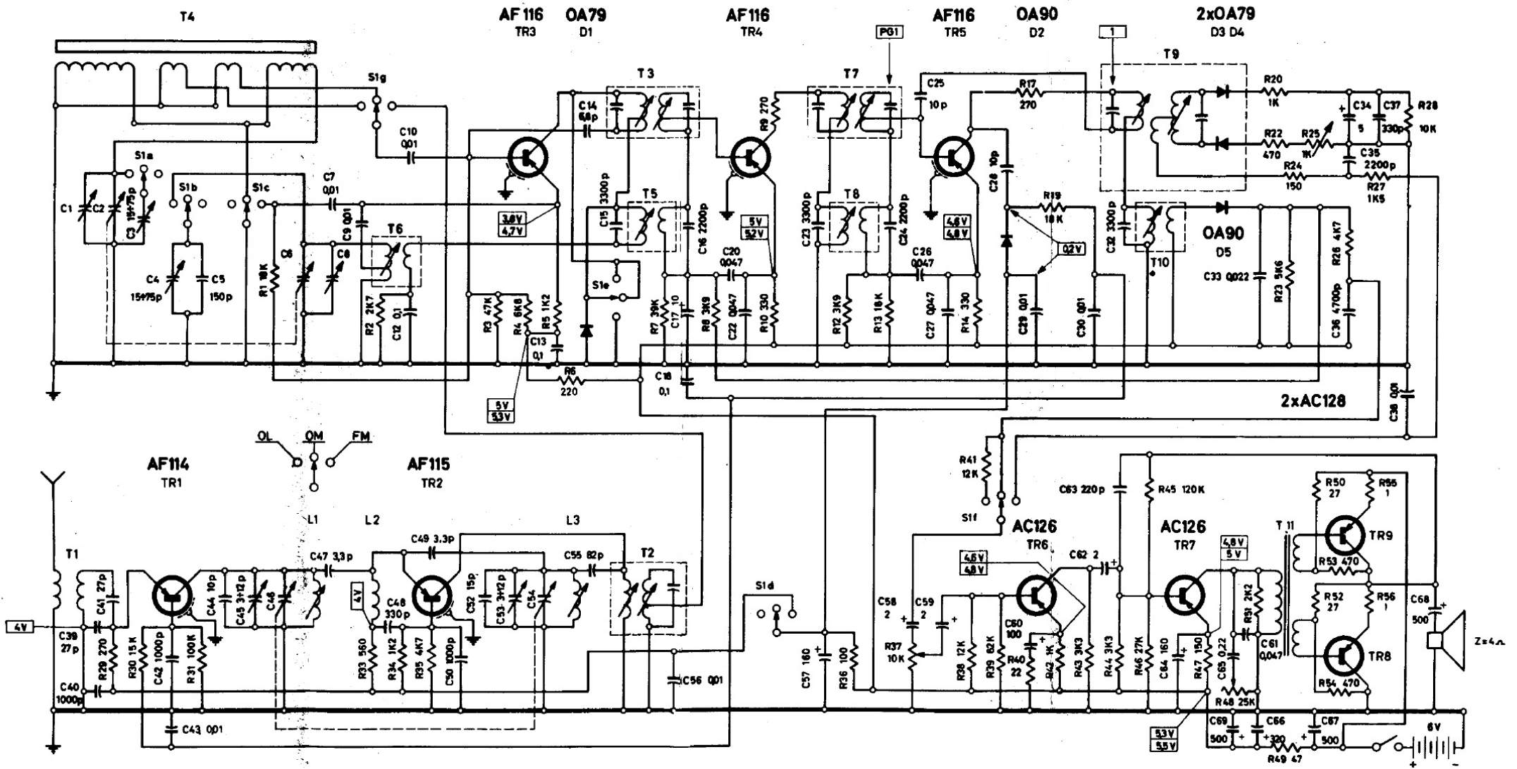
Tavola F — Schema di apparecchio radio a modulazione di ampiezza e di frequenza, a 9 transistor e cinque diodi (Voxson mod. 760).
